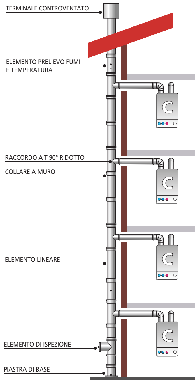
FIGURA 18 Schema canna fumaria di tipo C
